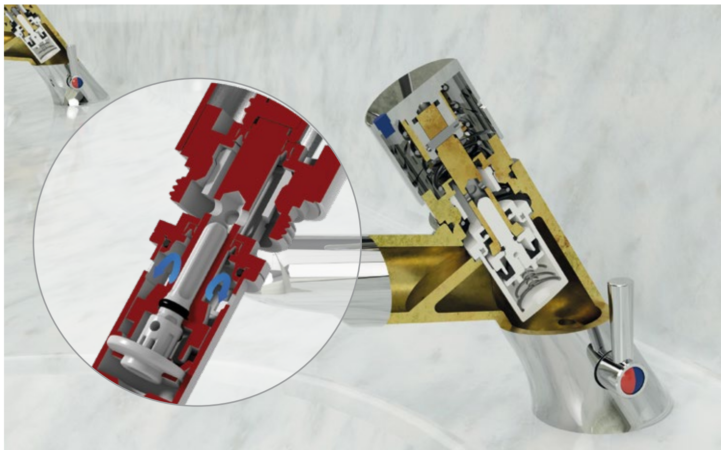
La chiusura è garantita anche in caso di blocco volontario del pulsante / Guaranteed flow stop in case of voluntary push button locking La fermeture est garanti même en cas de bloque volontaire du pussoir / El cierre está garantizado también en caso de bloqueo voluntario del pulsador
